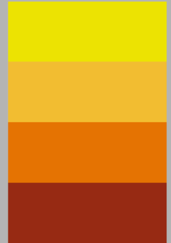
Analogus
